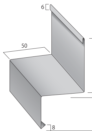
土台水切50
