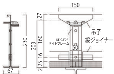
KDS-F25タイトフレーム
