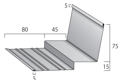
T型ジョイナー (カラー品対応)
