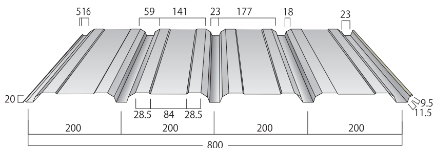
II型断面図（縦張・横張）
