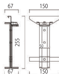
KDS-F50タイトフレーム
