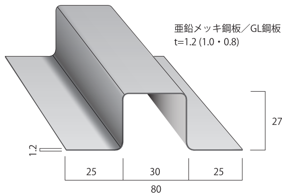
金属タルキ
