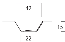
重ね部
