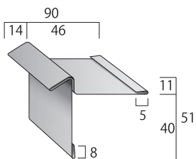
ケラバ唐草ER-23 e/レーフ型用
