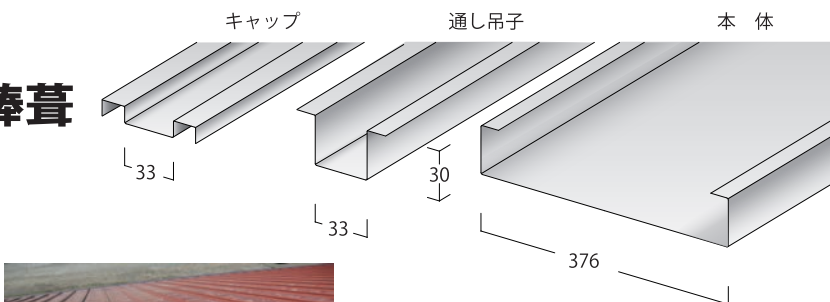
芯木無し瓦棒葺
