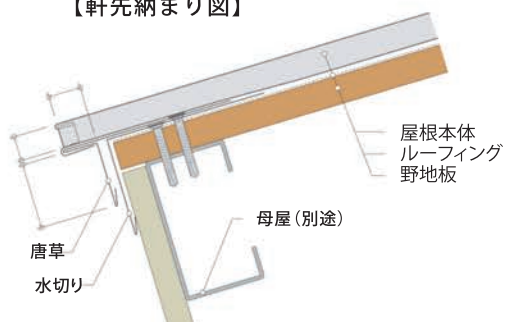
【軒先納まり図】
