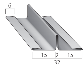
T型ジョイナー (カラー品対応)
