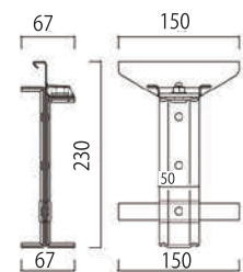
KDS-F25タイトフレーム
