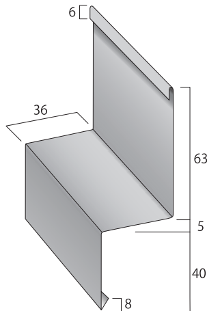
土台水切36
