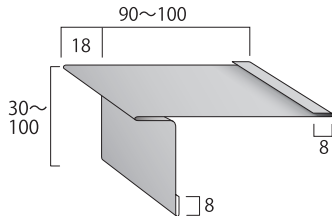
軒先唐草ER-32 e/レーフ型用
