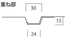
重ね部
