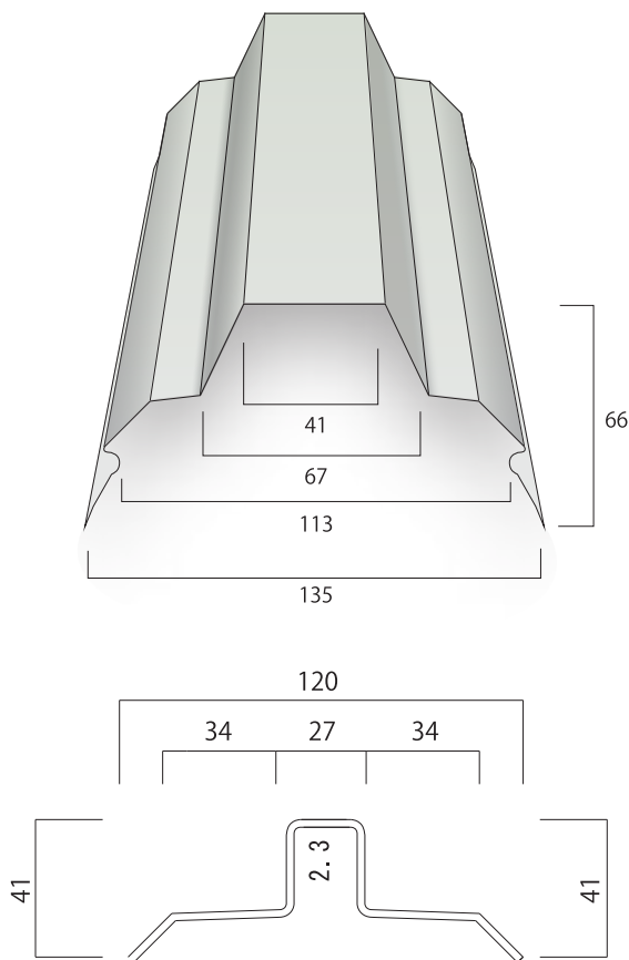
KR166ハゼキャップ
