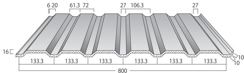
I型断面図
