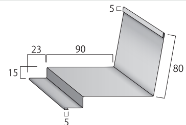
捨板
