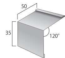
軒先水切
