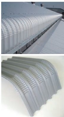
折下げ最低100mm以上、水上長さ最低1,200mm以上
