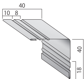
瓦棒唐草(R対応)
