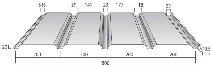
II型断面図（縦張・横張）
