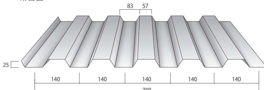
断面図
