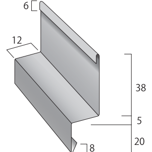
中間水切
