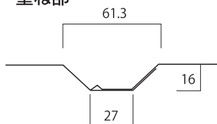
重ね部
