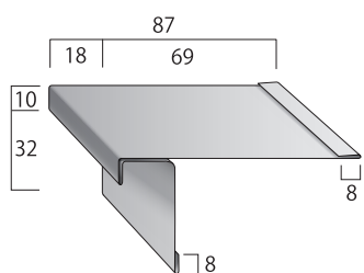
ケラバ唐草ER-23 e/レーフ型用
