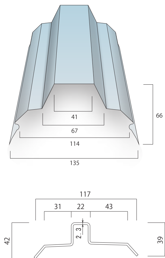
KR角ハゼ500(D160Ⅱ)ハゼキャップ
