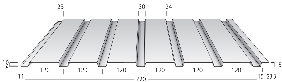
II型断面図（縦張・横張）
