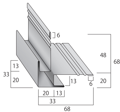
イカ頭出隅コーナー
