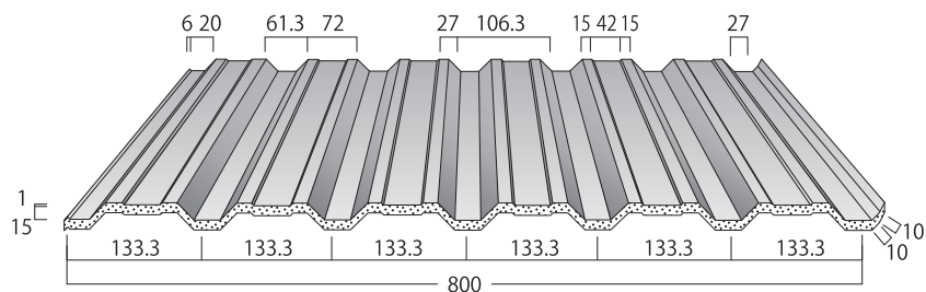
II型断面図
