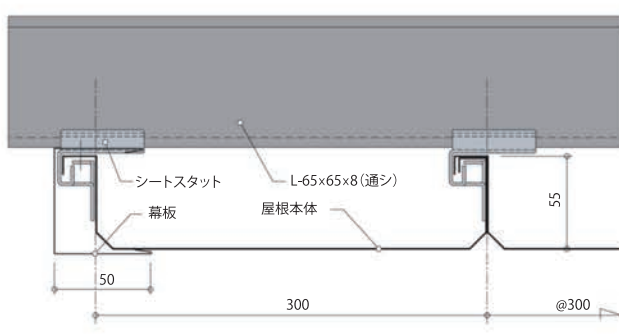
【ケラバ納まり図】
