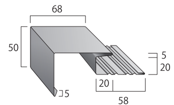
雨押え
