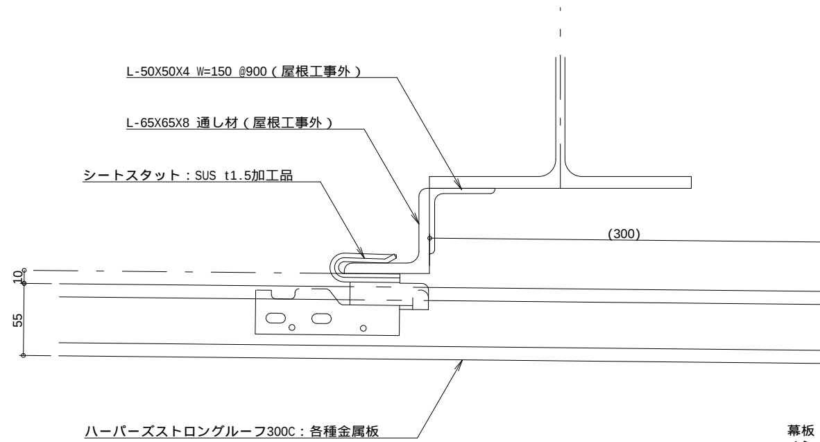
片棟詳細図
