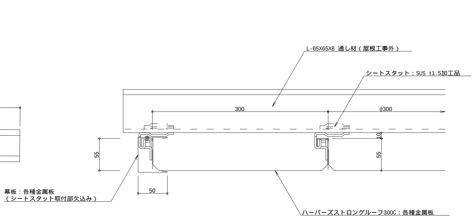
ケラバ詳細図
