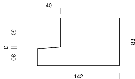
見切水切加工寸法
