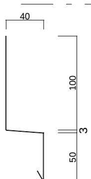
腰水切加工寸法
