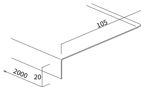
SUS-2B けらば力骨 t=0.8
