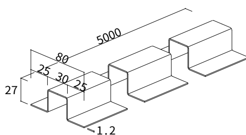
金属タルキ t=1.2
