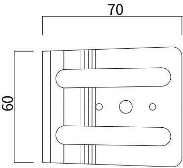
SUS・GL 吊子 t = 0.8
