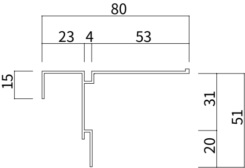
アルミけらば唐草 t = 1.5
