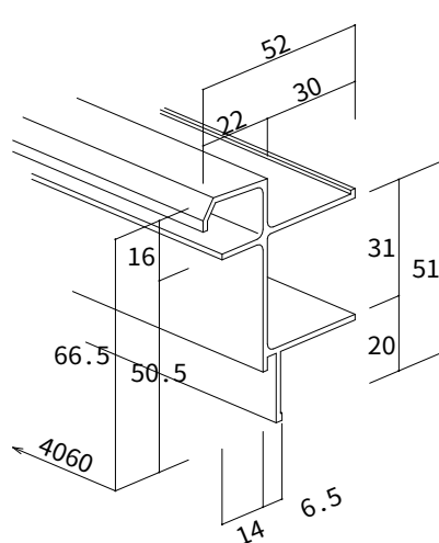
アルミ軒先唐草 (金属タルキ用) t=1.3
