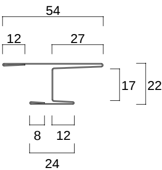
SPR - 400 (H型接続口ール成形品) L = 2000 ~ 3000
