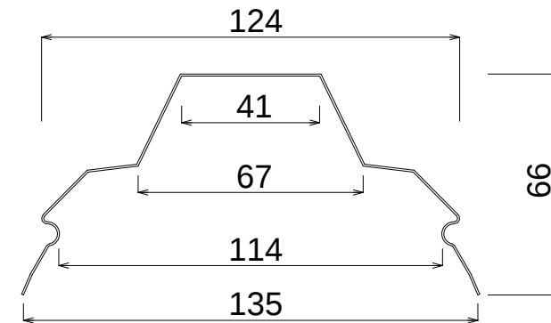
K R角ハゼ500 ( D 1 6 0 ) ハゼキャップ 板巾 = 2 2 7 mm
