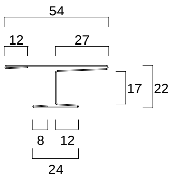
S P R - 4 0 0 ( H型接続口ール成形品 ) L = 2 0 0 0 ~ 3 0 0 0
