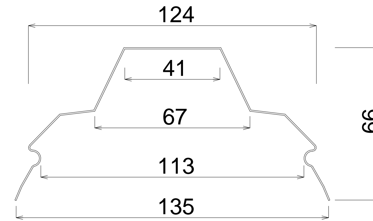
K R 1 6 6 ハゼ用・キャップ 板巾 = 2 2 7 mm
