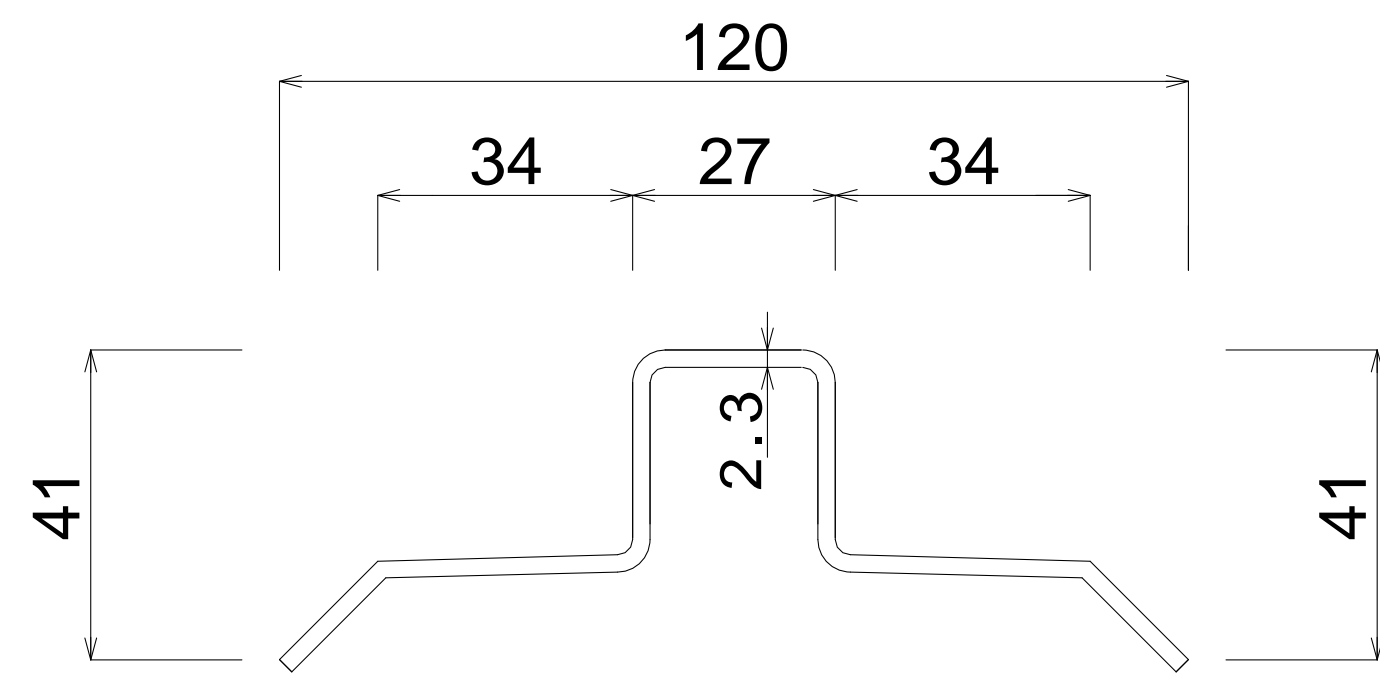
K R 1 6 6 ハゼ用・吊子W = 3 0
