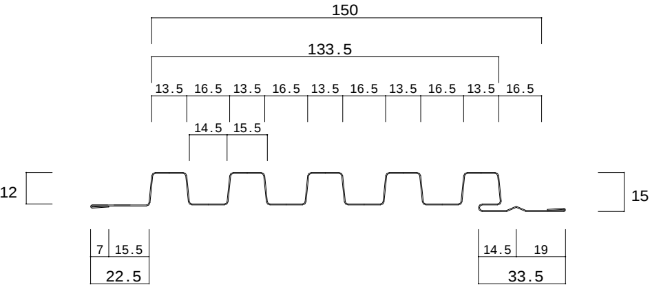
新リブスパン 1 5 0
