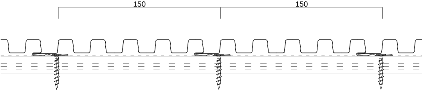
新リブスパン 1 5 0 ( 嵌合参考図 )
