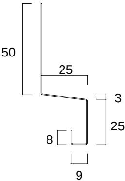
R S - 2 0 2 ( 中間水切接続 ) L = 2 0 0 0 ~ 3 0 0 0
