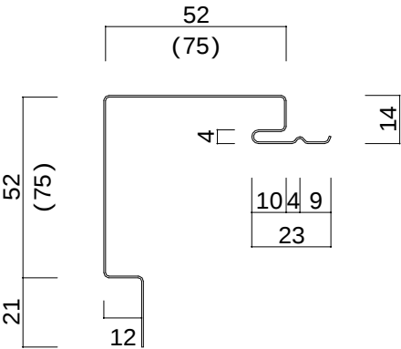
R S R - 3 0 3 ( 出 隅 ) L = 2 0 0 0 ~ 3 0 0 0
