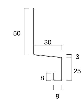
NK - 2 0 2 ( 中間水切接続 ) L = 2 0 0 0 ~ 3 0 0 0
