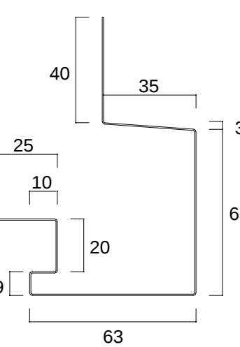
NK - 1 5 0 ( 天井正面接続 ) L = 2 0 0 0 ~ 3 0 0 0
