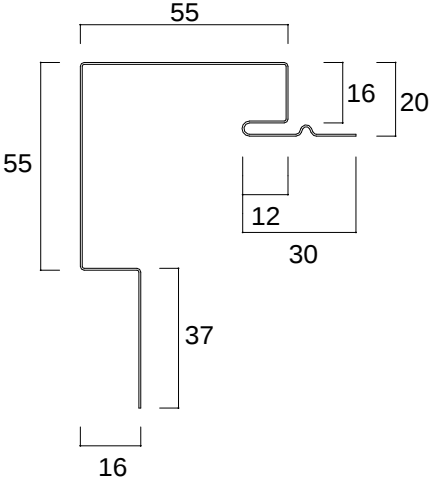
NKR - 3 0 3 ( 出 隅 ) L = 2 0 0 0 ~ 3 0 0 0
