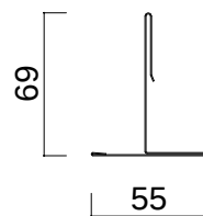
縦ジョイナー L = タイトスパン、- 60 mm
