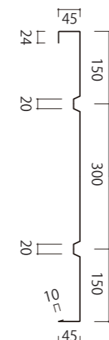
鼻隠しH600
