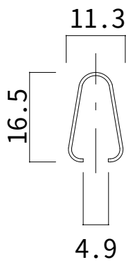
アーチルーフキャップ
