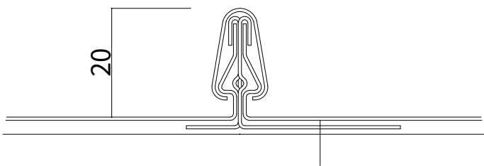
葺方向左→右図 （右→左でも可）
