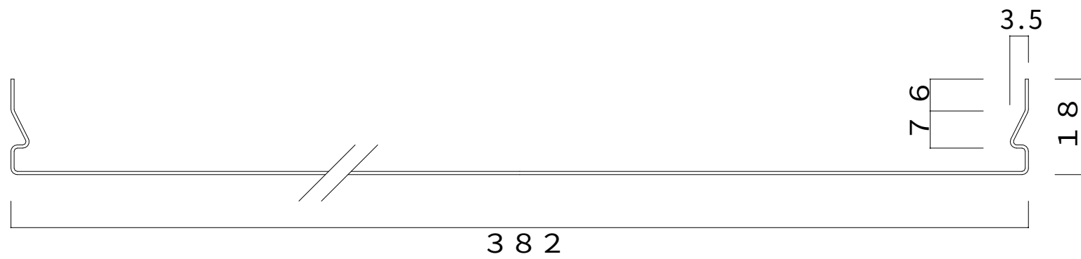
アーチルーフ溝板
