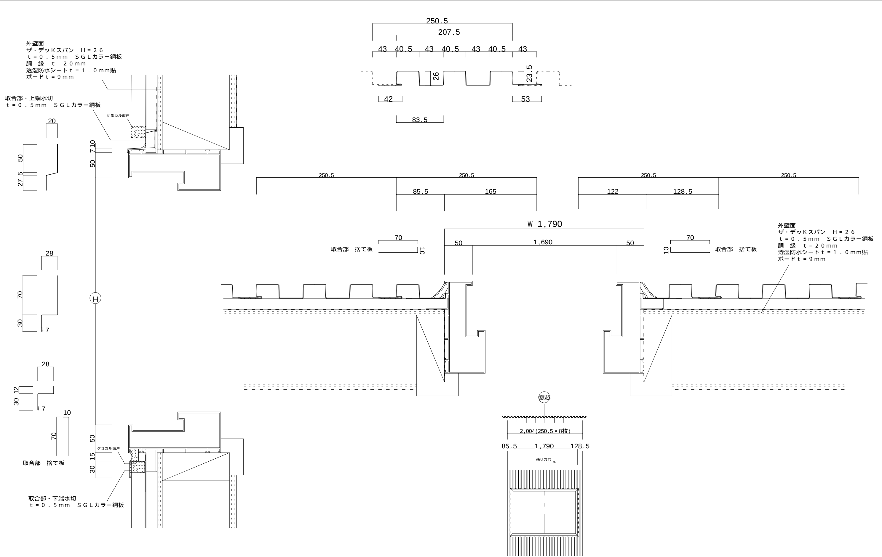
割付図 1/30
