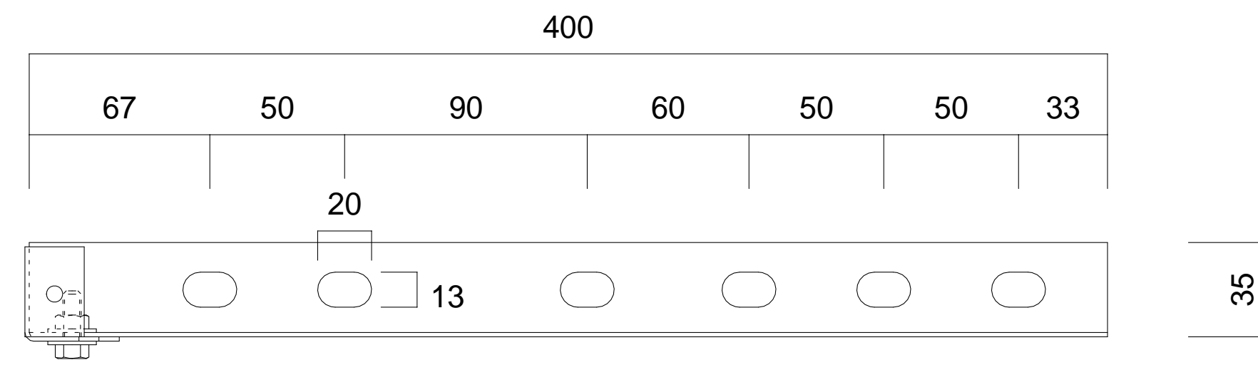
鼻隠し DX300 取付金物
