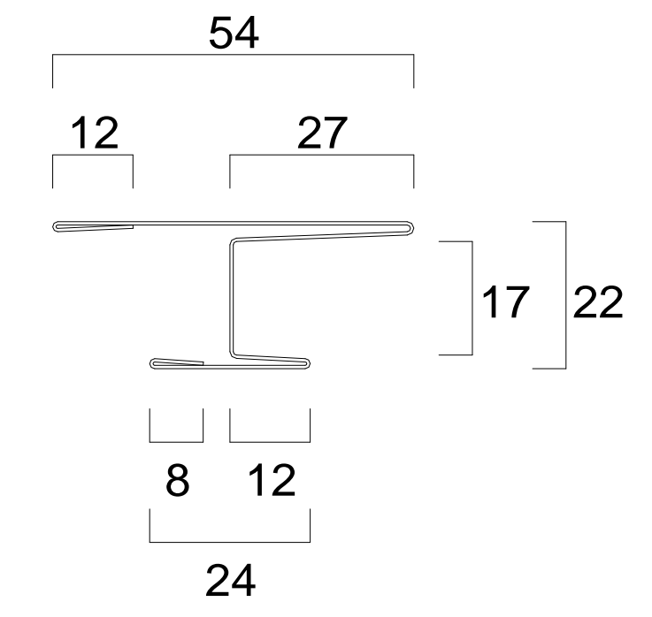
SPR-400 (H型接続口ール成形品) L = 2000 ~ 3000
