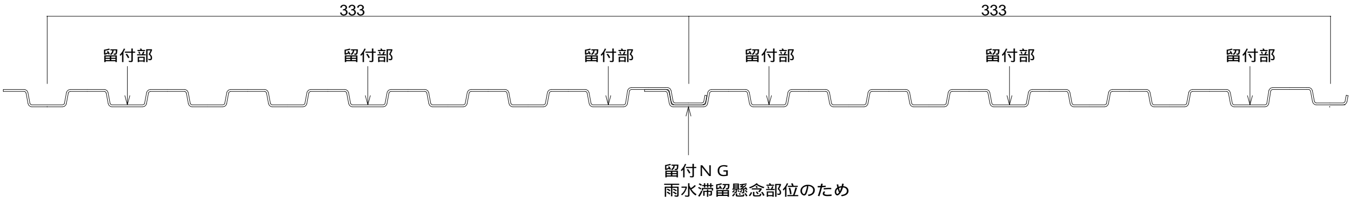
ファスナー類留付位置（参考）
