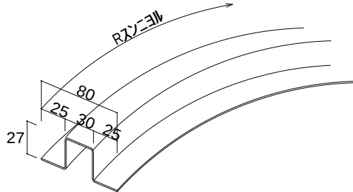
特殊金属タルキ t = 1 . 2
