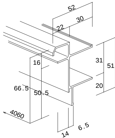
SUS - 2 B 軒先力骨 (直葺用) t = 0 . 8
