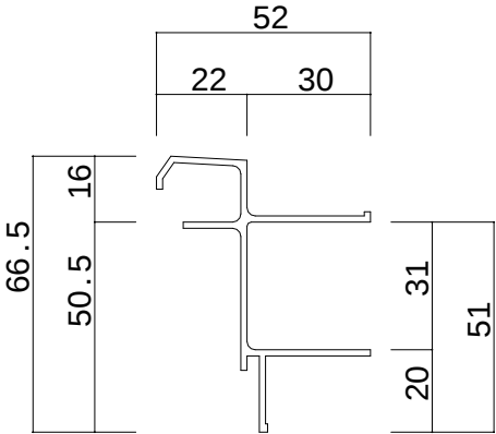
アルミ軒先唐草（金属タルキ用）t = 1 . 3
