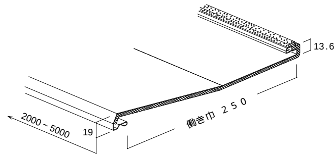
ロイヤル横葺 2 5 0 継手カバータイプ本体形状
