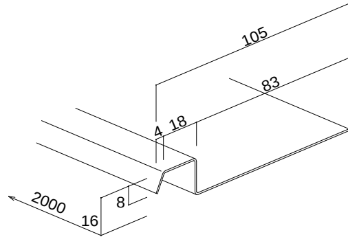
SUS - 2 B 軒先力骨 (直葺用) t = 0 . 8
