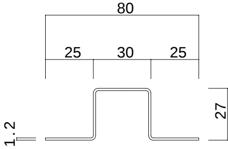
金属タルキ t = 1 . 2
