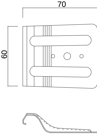
S U S ・ G L 吊子 t = 0 . 8
