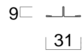
横ジョイナー L = 995
