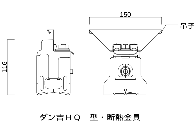
ダン吉HQ 型・断熱金具 上記断熱金具 : (株) サカタ製作所製品
