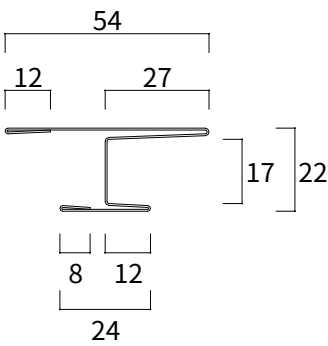
SPR-400 (H型接続ロール成形品) L=2000~3000
