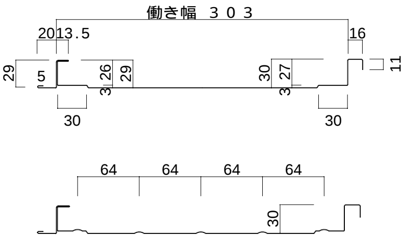
DKライン303(H30型) 縦リブ仕様フラット品のみ
