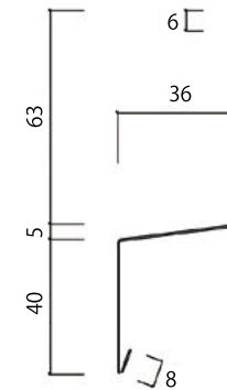
イカ頭出隅コーナー
