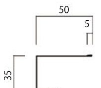
軒先水切
