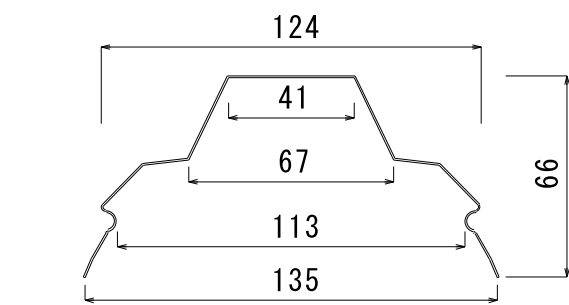
KR166ハゼキャップ
