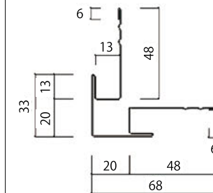
イカ頭出隅コーナー
