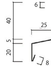
土台水切25
