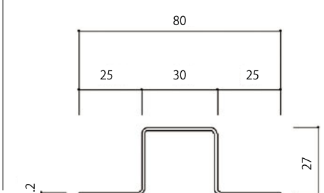
金属タルキ
