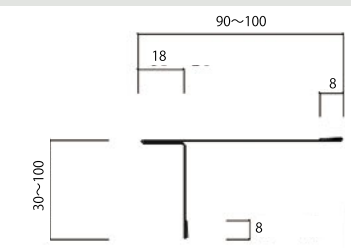
T型ジョイナー(カラー品対応)
