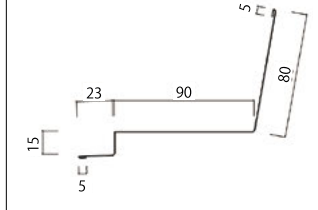
瓦棒唐草(R対応)
