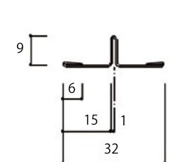
T型ジョイナー(カラー品対応)
