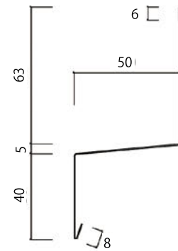
けらば水切
