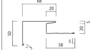
けらば水切
