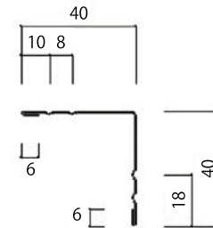
棟包み
