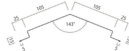
eルーフI型用軒先唐草ER-32
