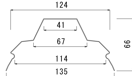
KR角ハゼ500(D160II)ハゼキャップ
