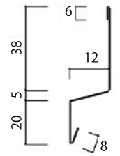
中間水切
