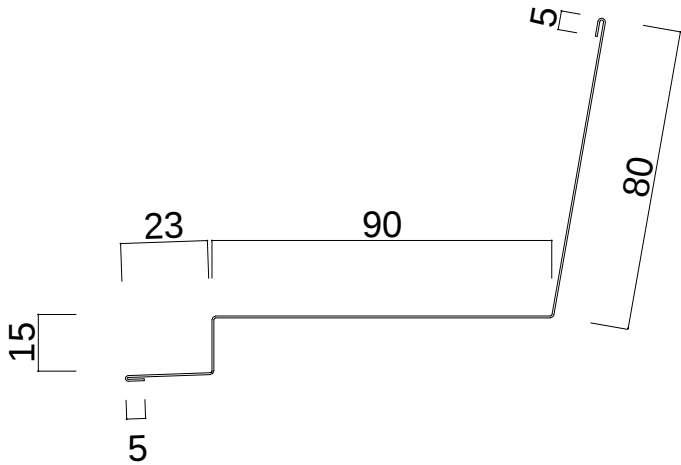
Y A R 雨 押 え ( L = 1 , 8 2 9 mm )
