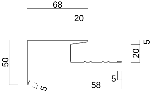
Y K R けらば水切 ( L = 1 , 8 2 9 mm )
