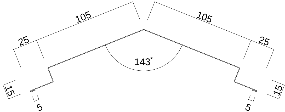
M R R 棟 包 み ( L = 1 , 8 2 0 mm )
