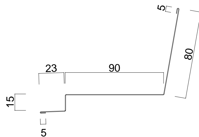
Y A R 雨 押 え ( L = 1 , 8 2 9 mm )
