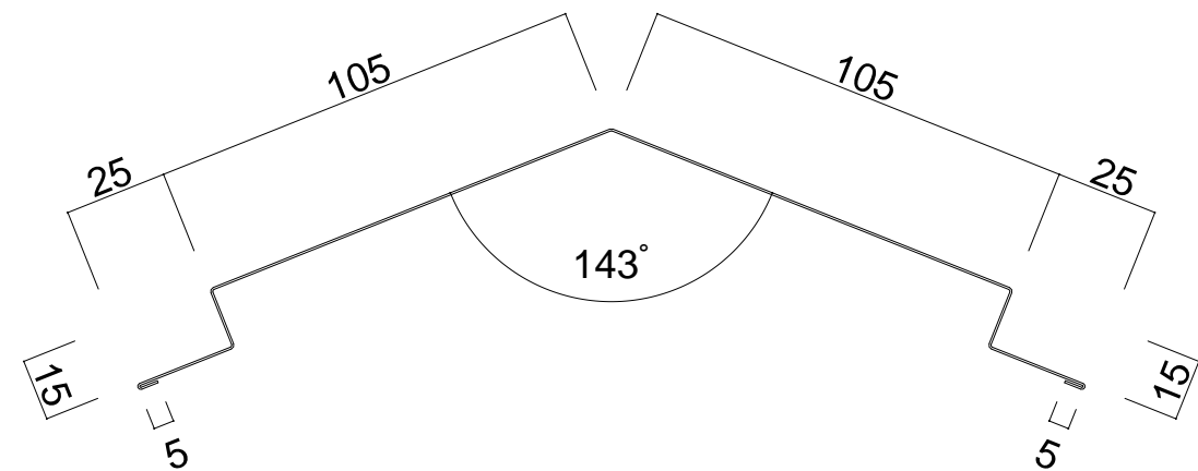
M R R 棟 包 み ( L = 1 , 8 2 0 mm )
