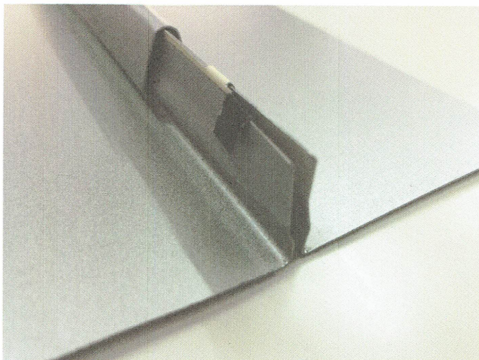
①立上凸部をフラットにすると差込可能です
