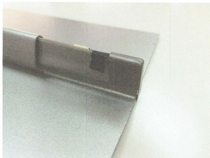
②差込んだ状態（軒先掴み込み前の先付け取付のみ可能）
