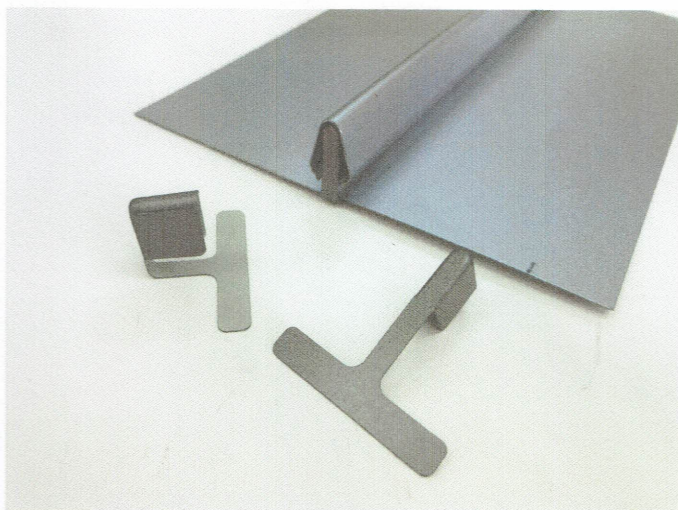
⑥軒先サン魅せる部材での軒先仕舞（化粧軒先提案）
