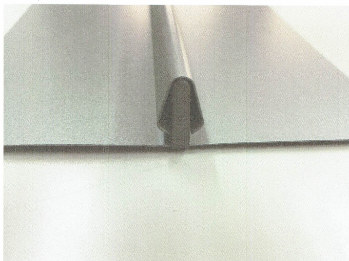
③キャップ先端合せ状態仕舞1
