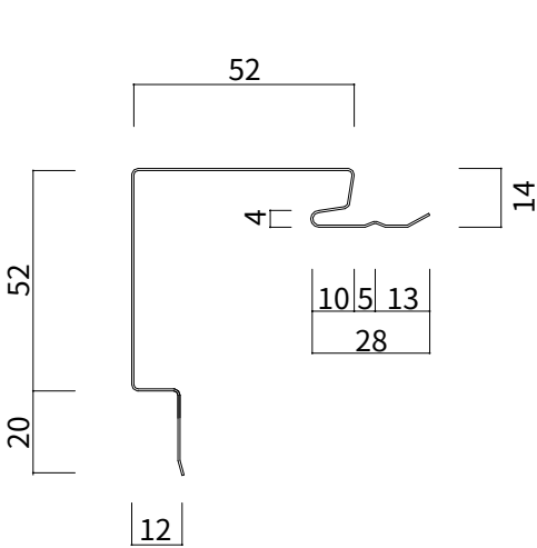
SPR116 (出隅) L=2000~3000
