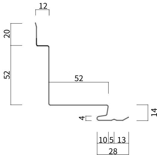
SPR116 (入隅) L=2000~3000
