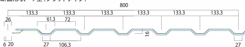
断面形状 II型(リップタイプ)
