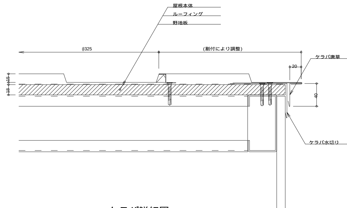
ケラバ詳細図
