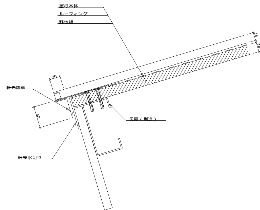
軒先詳細図
