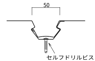
B L ウォールジョイント
