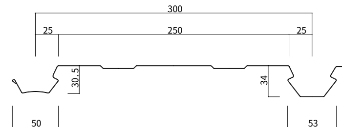
B L ウォール断面図
