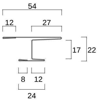
SPR - 400 (H型接続口ール成形品) L = 2000 ~ 3000
