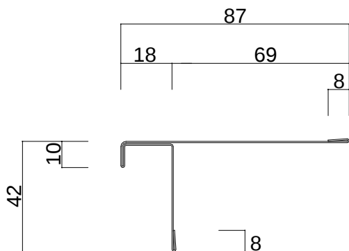
鋼板製（ e ルーフ 型 ・ 型兼用 ） けらば唐草 E R - 2 3
