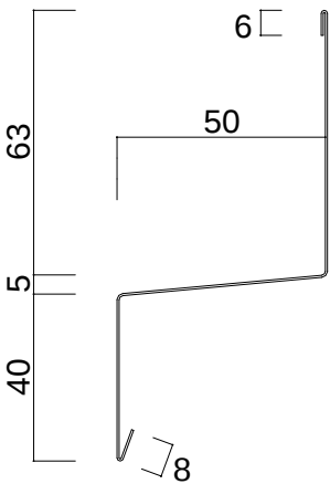
土台水切 5 0 （ L = 3 , 0 3 0 mm ）
