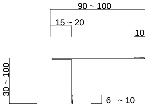
R 対応鋼板製 けらば唐草
