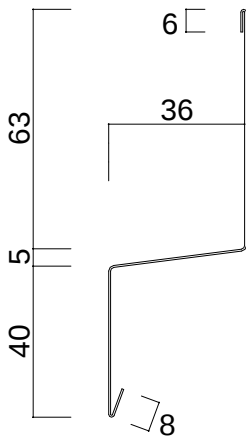
土台水切 3 6 （ L = 3 , 0 3 0 mm ）
