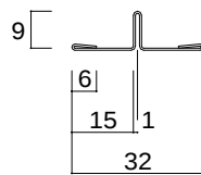
T型ジョイナー（ L = 3 , 0 3 0 mm ）
