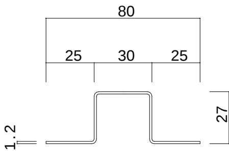
金属タルキ t = 1 . 2
