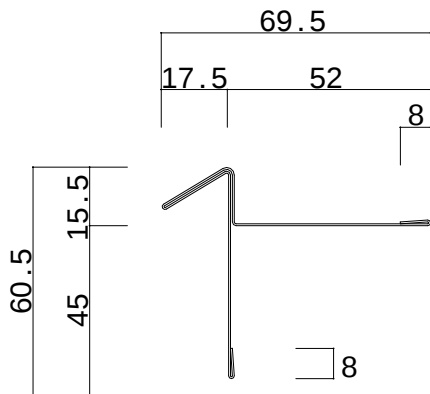
鋼板製（ e ルーフ 型用 ） 軒先唐草（木造用） E R - 3 3
