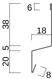
中間水切 1 8 （ L = 3 , 0 3 0 mm ）
