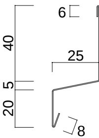
土台水切 2 5 （ L = 3 , 0 3 0 mm ）
