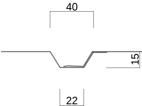
重ね部形状
