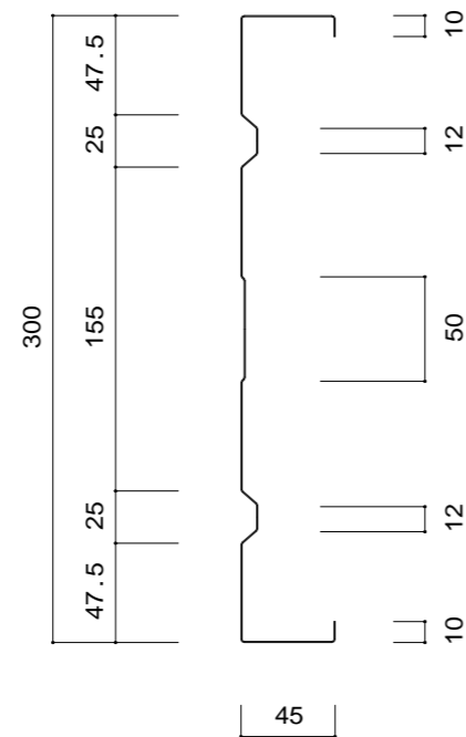
鼻隠しH300 (リップ付き)
