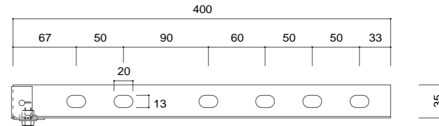
鼻隠しH300取付金物 (佐野庄製品)
