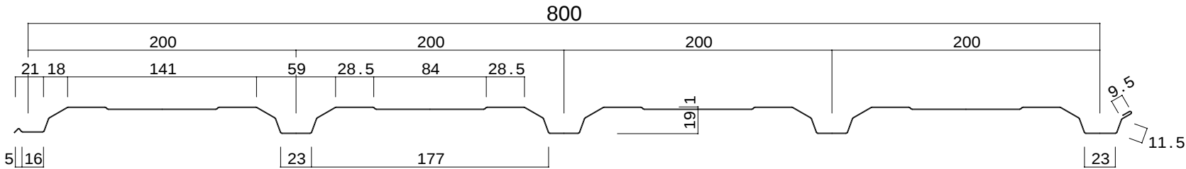
KW800N 型（リブ付） 縦張り・横張り
