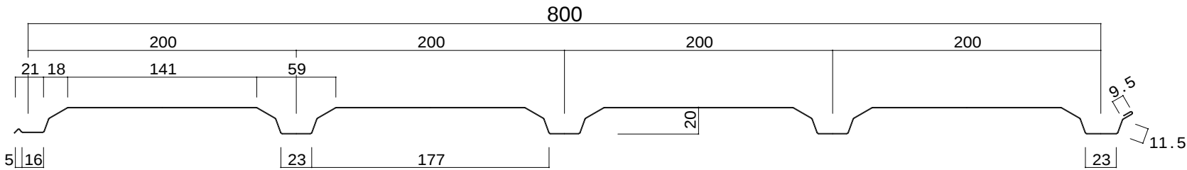
KW800N 型（リブ無し） 縦張り
